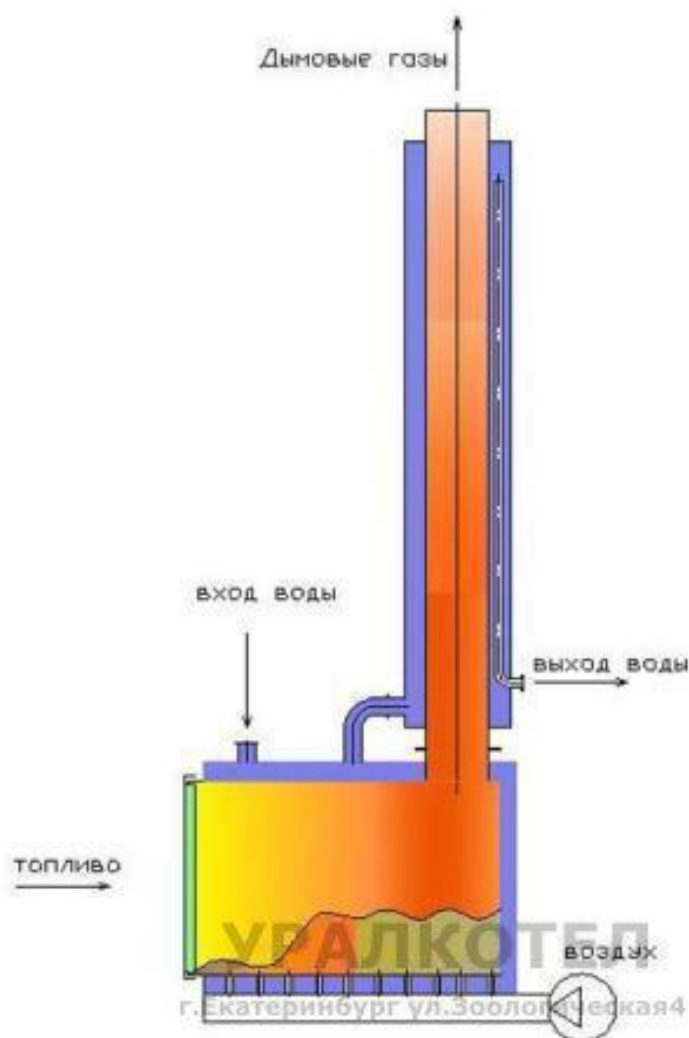
Рисунок 2.1 – Принципиальная схема котла КВСрд 0,5
